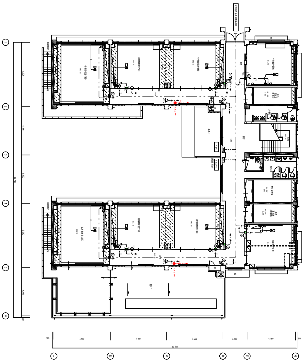
2階平面図 1/100
