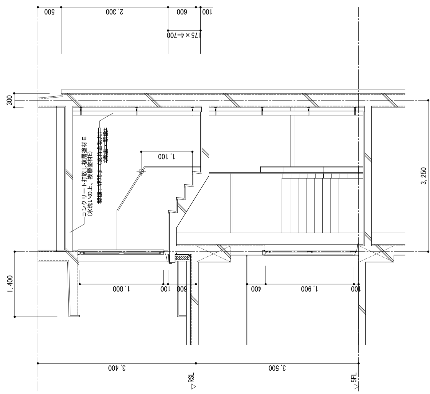
屋上階段詳細図 S-1/50
