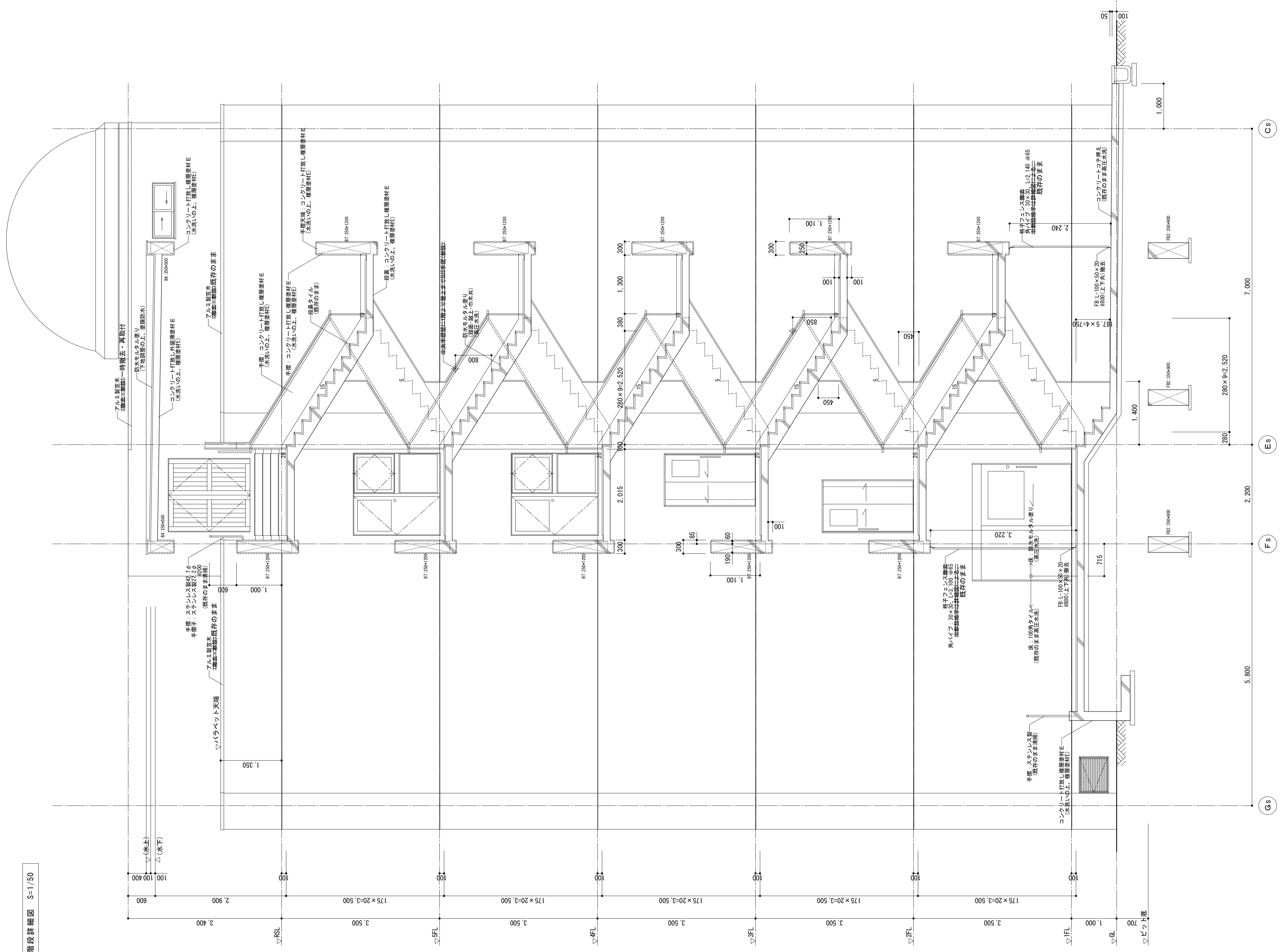
化粧リブ詳細図 S-1/10
